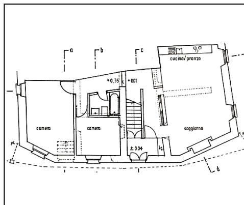
Grundriss der Parterrewohnung
